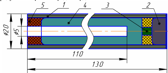
Рис 1 - схема двигателя РД1-30-5
