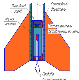
Рис. 4 - порядок запуска.
