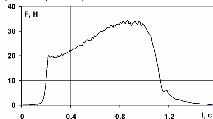
Рис 2 - График изменения тяги двигателя РД1-30-5
